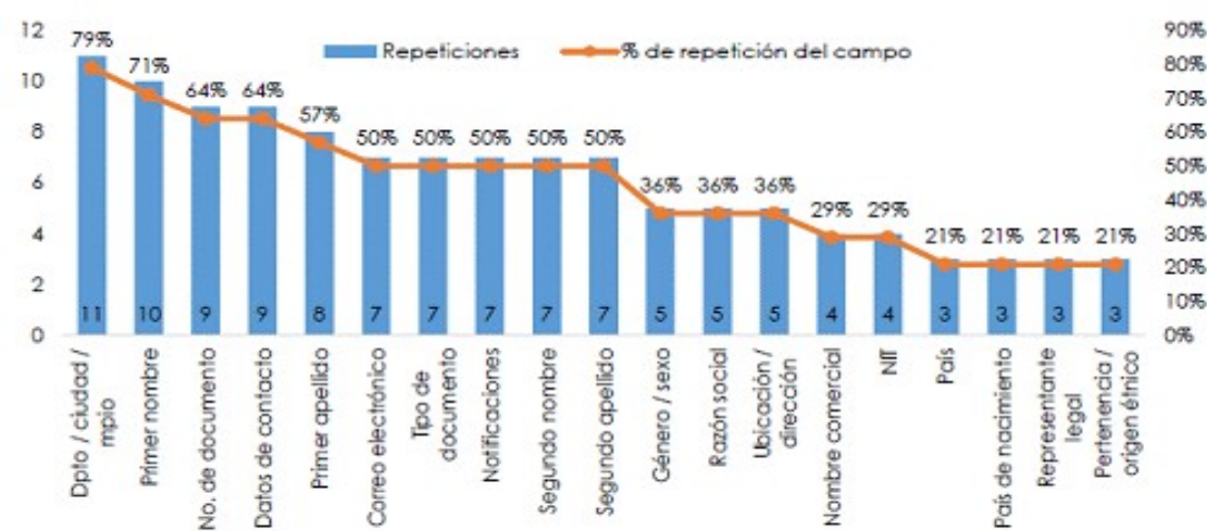
Gráfico 13. Índice de redundancia de campos de registros
